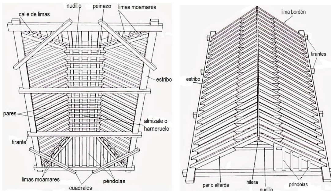
Figura 16. Ejemplo de cubierta realizada con estructura de par y nudillo. Tomado de https://www.glosarioarquitectonico.com/glossary/armadura/ el 18 de noviembre del 2022
