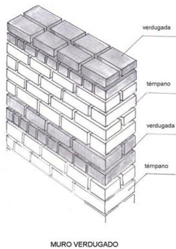
Figura 17. Ejemplo de un muro verdugado. Tomado de https://www.google.com/search?q=muros+verdugados
