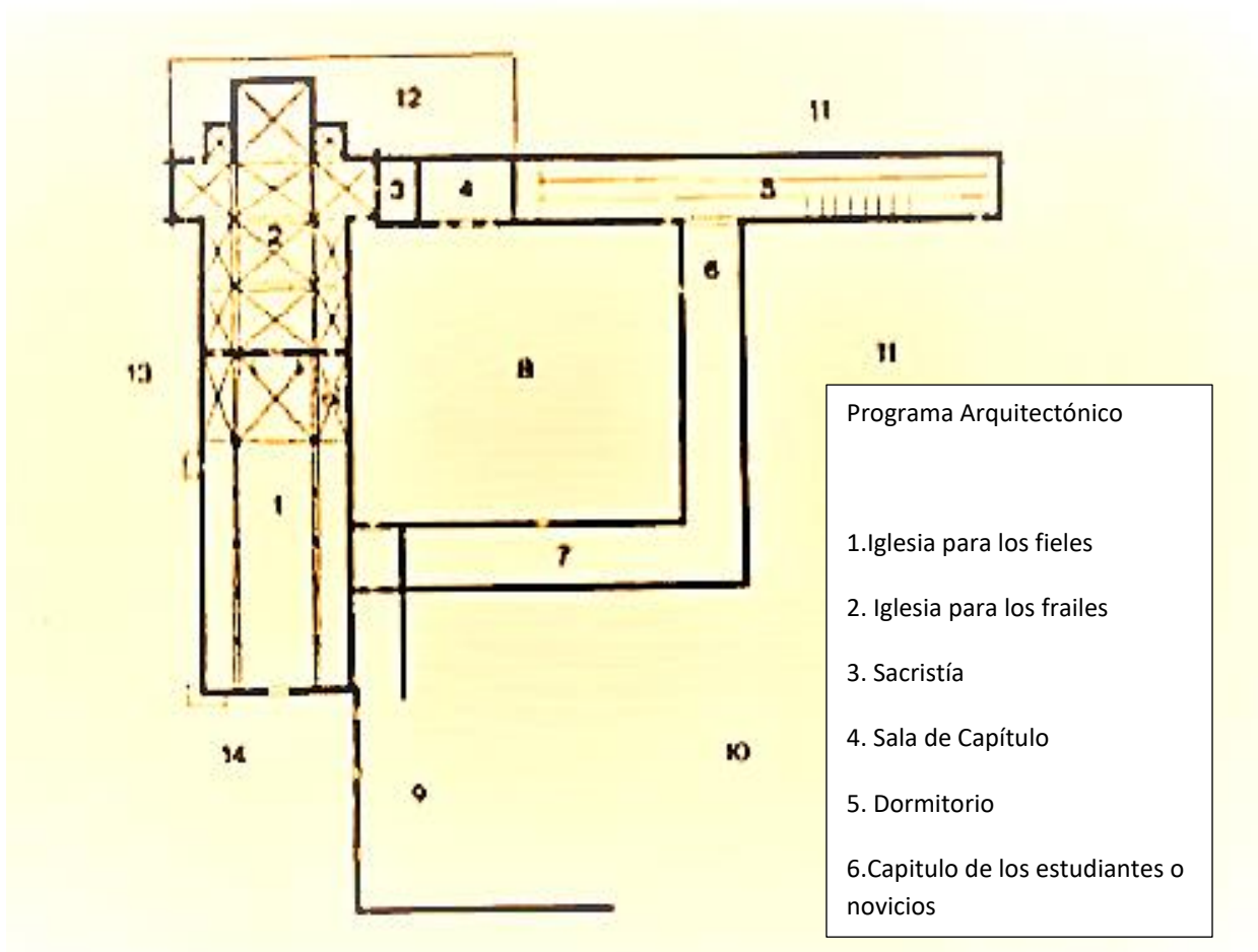
Figura 14. Planta del Convento dominico de Bolonia en el siglo XIII. Tomado de Ovando, op.cit. , p. 57
